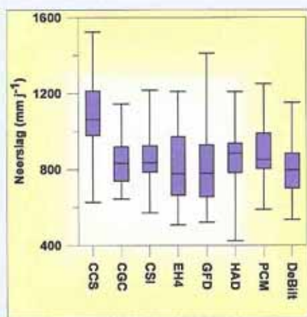
Afb. 4: Jaarlijkse (links) en maandelijkse (rechts) neerslagverwachtingen voor de periode 2035-2064 volgens de zeven klimaatmodellen. De maandelijkse waarden (rechts) zijn weergegeven als percentages van de jaarlijkse gemiddelde neerslag. Waarden van De Bilt zijn voor de referentieperiode 1961-1990.
