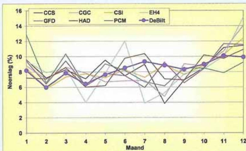
Afb. 4: Jaarlijkse (links) en maandelijkse (rechts) neerslagverwachtingen voor de periode 2035-2064 volgens de zeven klimaatmodellen. De maandelijkse waarden (rechts) zijn weergegeven als percentages van de jaarlijkse gemiddelde neerslag. Waarden van De Bilt zijn voor de referentieperiode 1961-1990.
